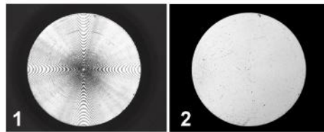
1: 金屬切剖面以環形光源照明效果 2: 金屬切剖面以半球形光源照明效果
